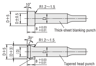
[Fig. 3] Punch shape
