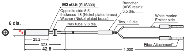
23-D E32-C41 1M (No Cutting) + E39-F3B
